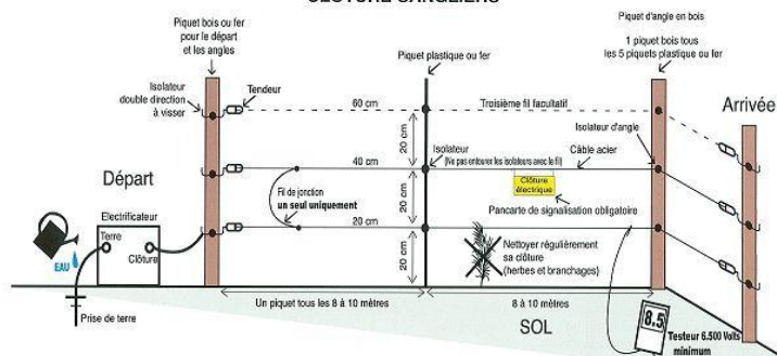
CLÔTURE SANGLIERS
