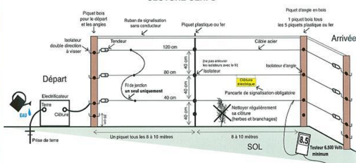
CLÔTURE CERFS
